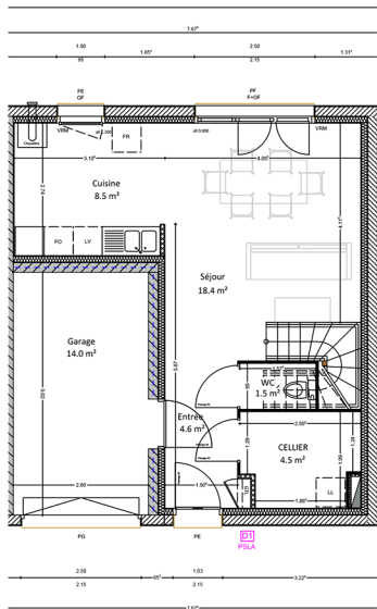
PLAN RDC
